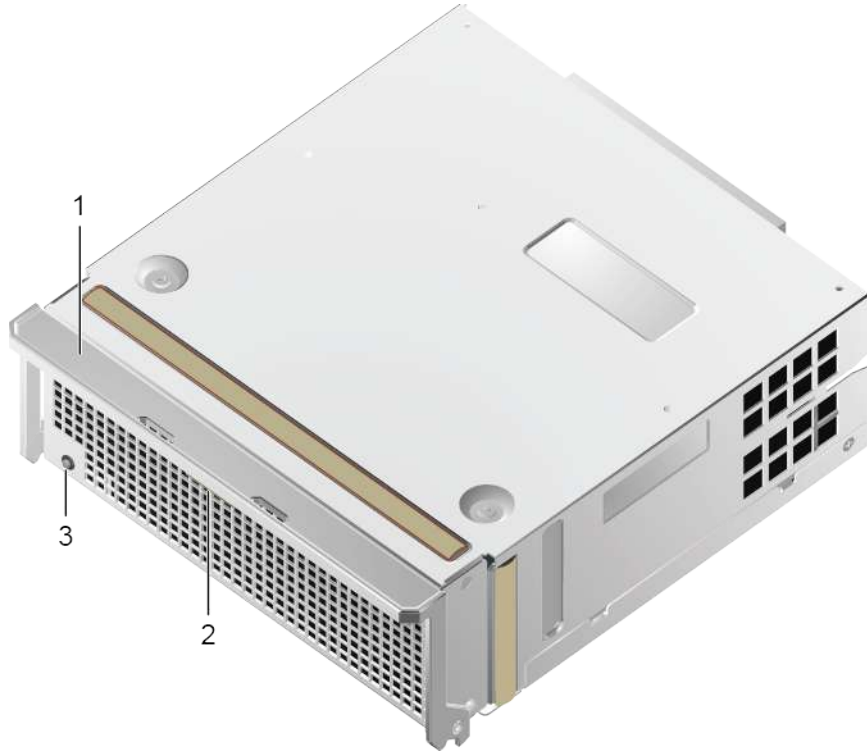
Figure 4-40 Fan module
